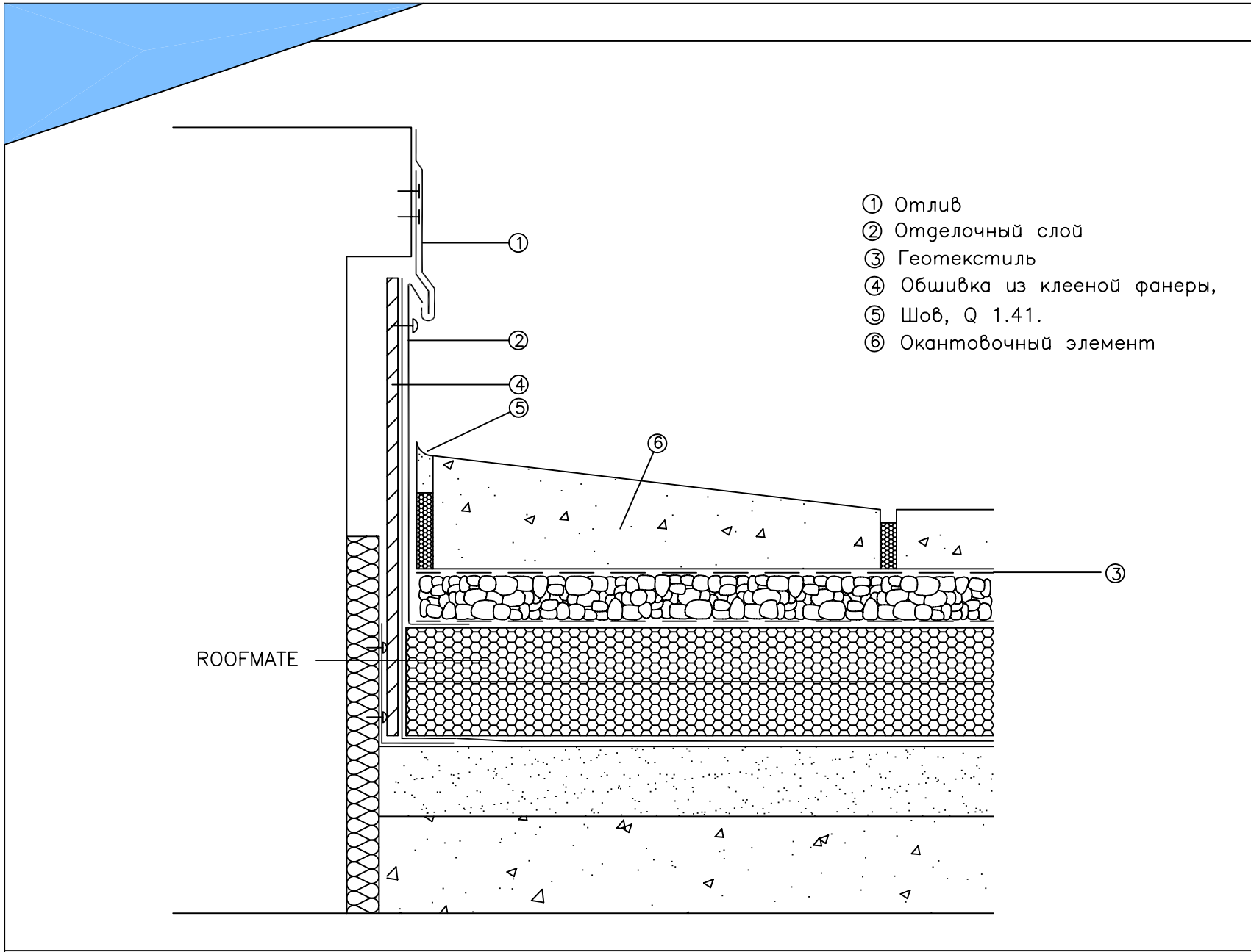
Рисунок Примыкание к стене
